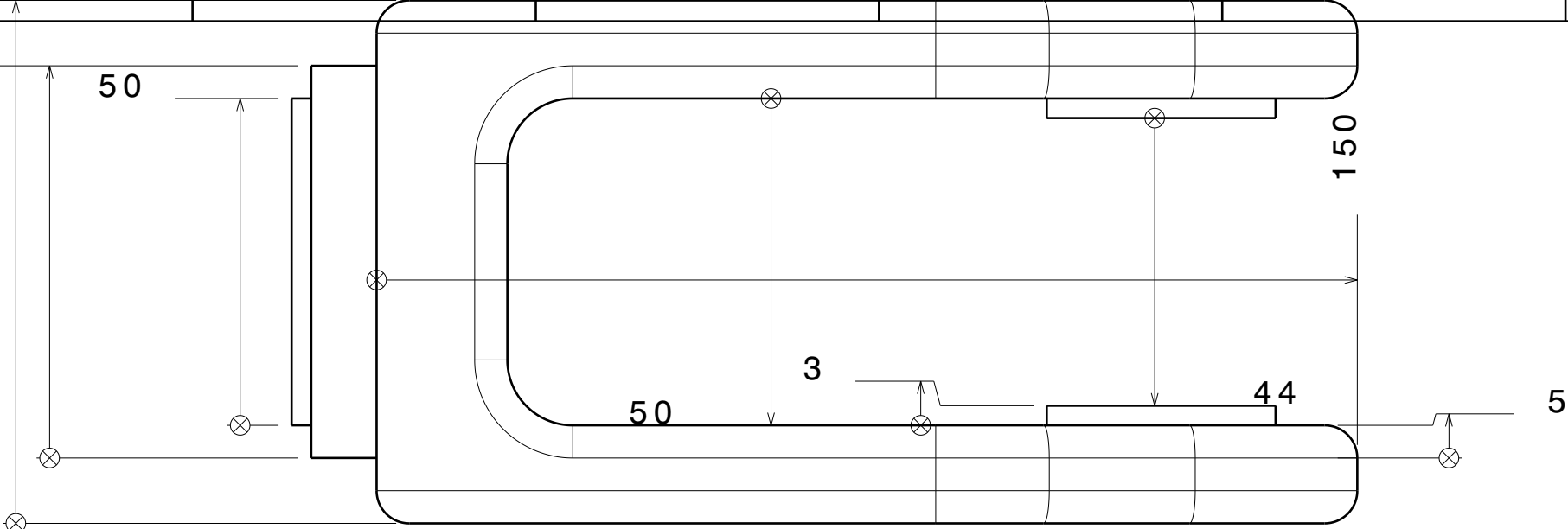
Bottom view Scale: 1:1
